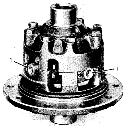
Fig. 6.2 I. CROSS PINS
